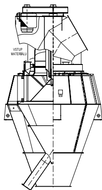
Воздушный сепаратор в исполнении LTR-M
